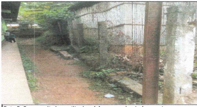
Foto 5: Se necesita la sustitucion del muro perimetral por extremo deterioro del mismo y es riesgoso para la seguridad de los niños en la escuela.
