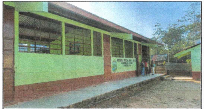
Foto 4: Se ve la necesidad de colocar canales al modulo 1, ya que en tiempo de invierno perjudica la acumulacion de agua que baja de las laminas al patio de la escuela, llevandose la tierra.
